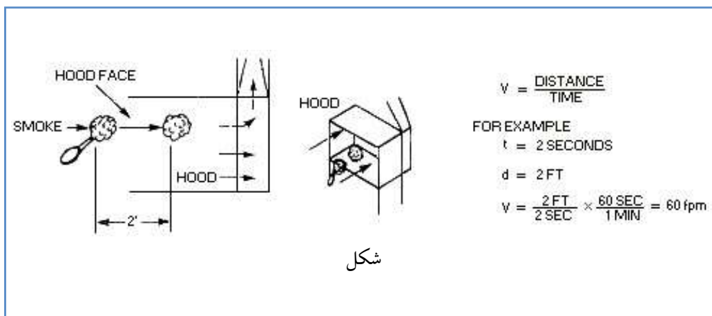
شکل ۳- هود میزی مخصوص لحیم کاری
